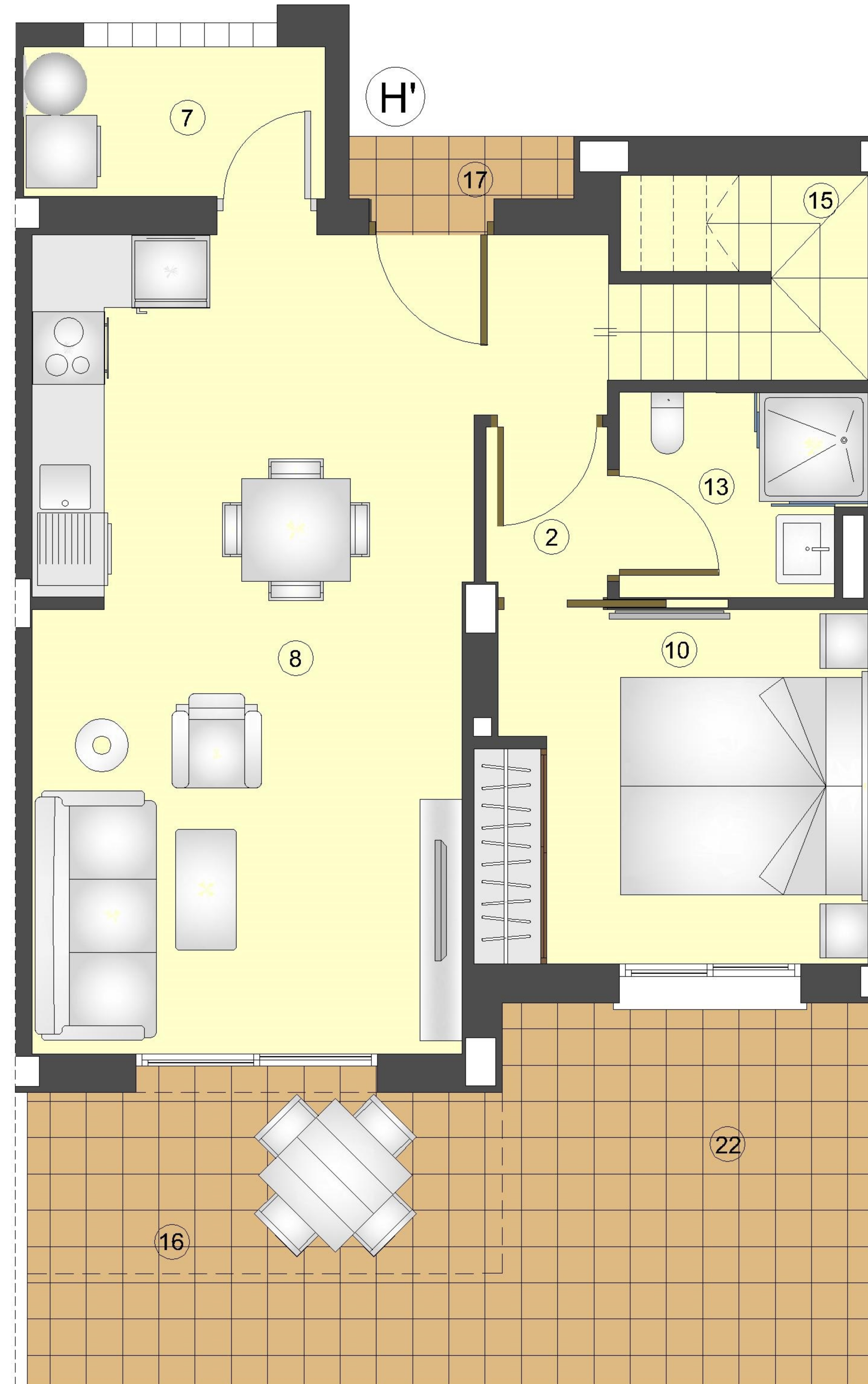
PLANTA BAJA
